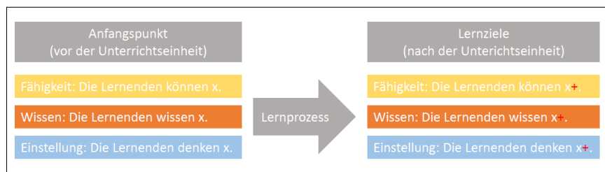
Abb. 2 Lernzielfelder
